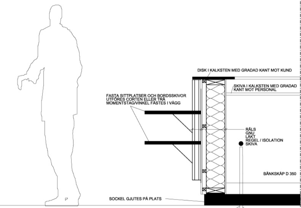
DETALJ 1 1:10
