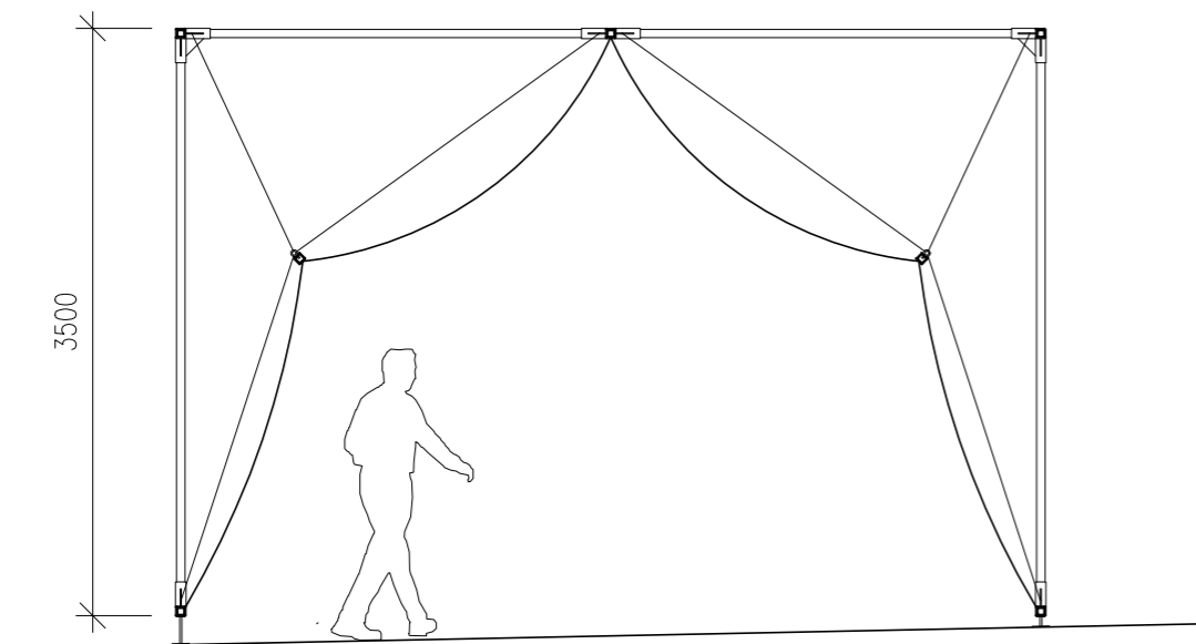
SEKTION
