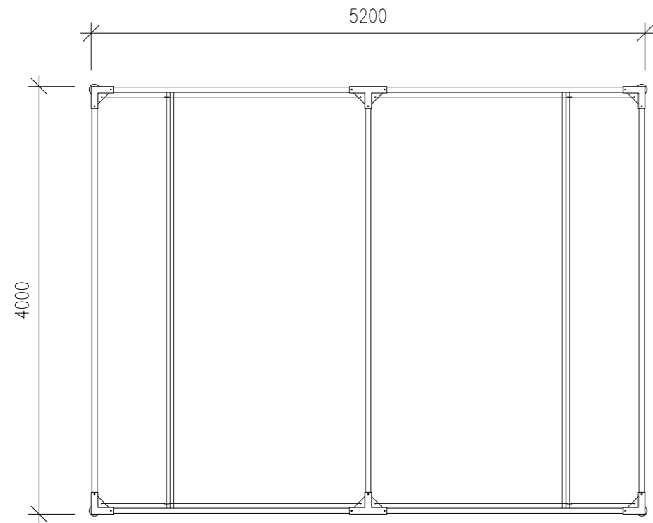
TAKPLAN
