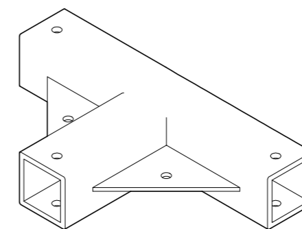
DETALJ MITTPROFIL
