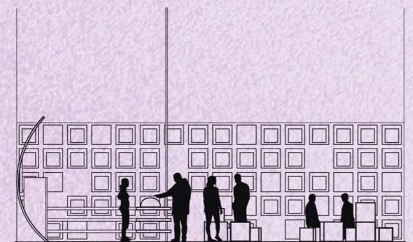
Sektion A:A
